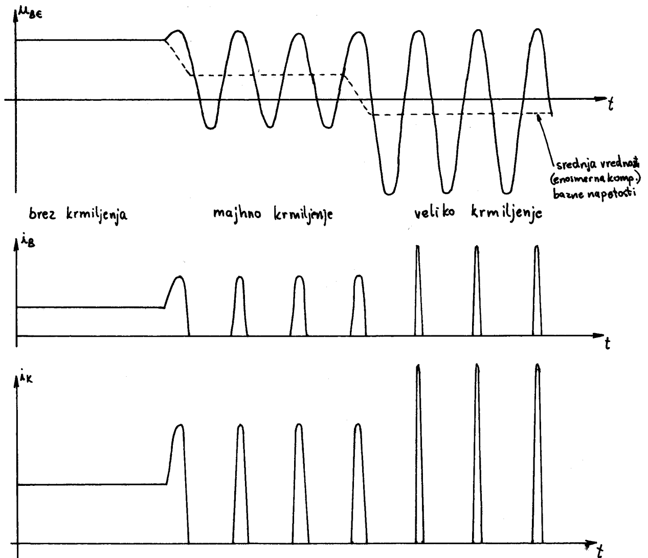
Delovanje tranzistorske množilne stopnje
