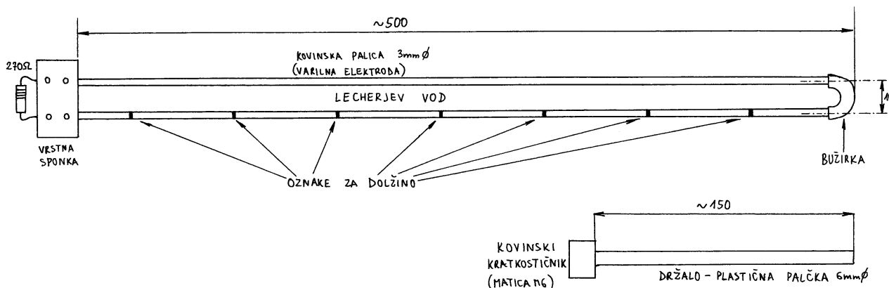
Slika 2 - Praktična izvedba Lecherjevega voda
