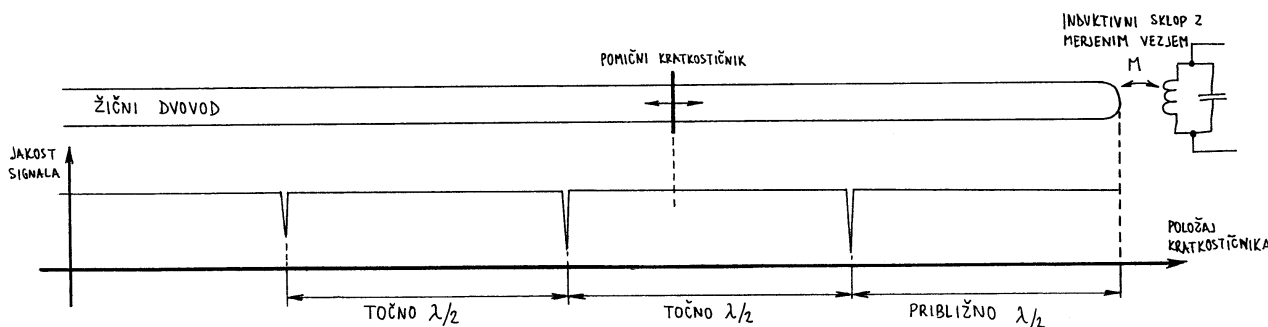
Slika 1 - Delovanje Lecherjevega voda
